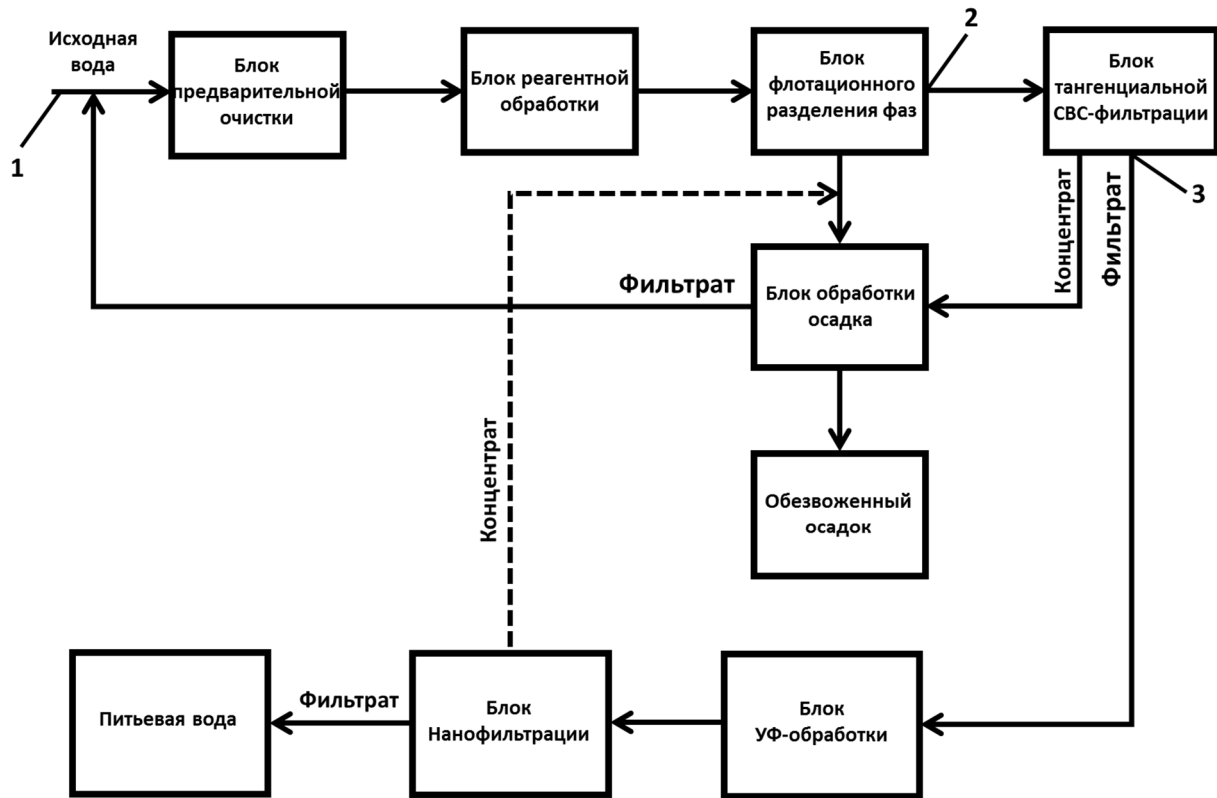
Рисунок 2 – Принципиальная схема блоков очистки воды
